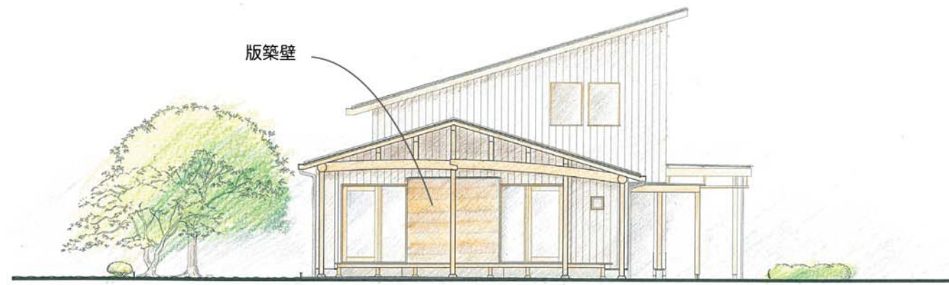
東立面図
